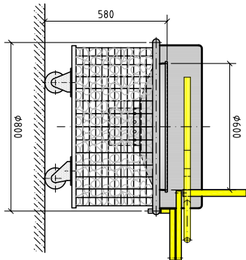
STONEHENGE III fahrbar Art. Nr. 00-660
