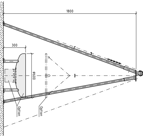
KARUGA II Art. Nr. 00-910
