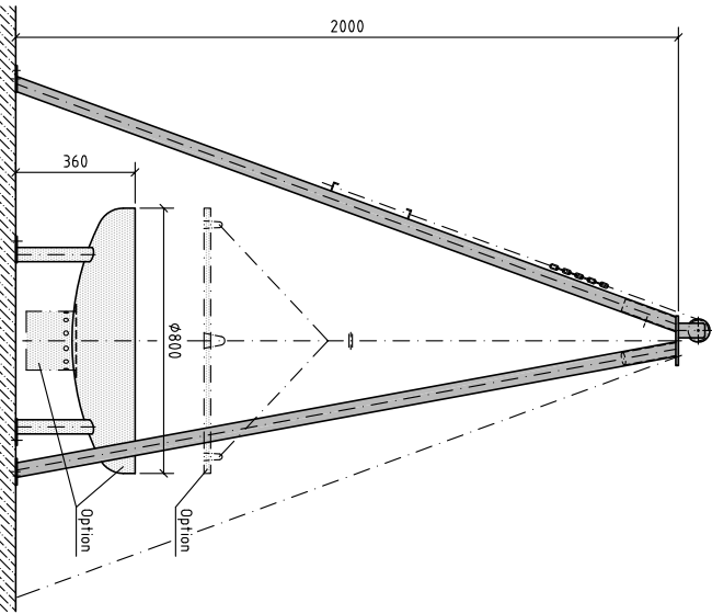
KARUGA I Art. Nr. 00-900
